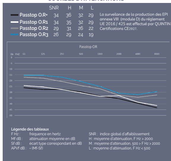
COURBES D'ATTENUATIONS
